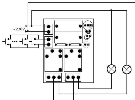
Rys. 2. Schemat podłączenia z wieloma przyciskami i żarówkami
