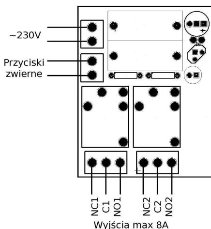
Rys. 1. Wprowadzenia przełącznika 2xON/OFF
