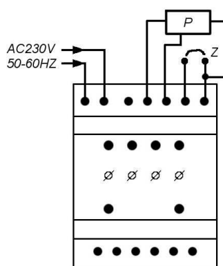
Rys. 5. Przykładowa konfiguracja z czujnikiem ciśnienia
