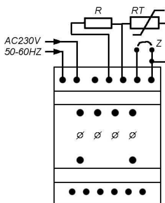
Rys. 4. Przykładowa konfiguracja z termistorem do pomiaru temperatury
