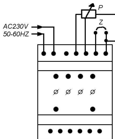
Rys3. Przykładowa konfiguracja z potencjometrem jako czujnikiem.
