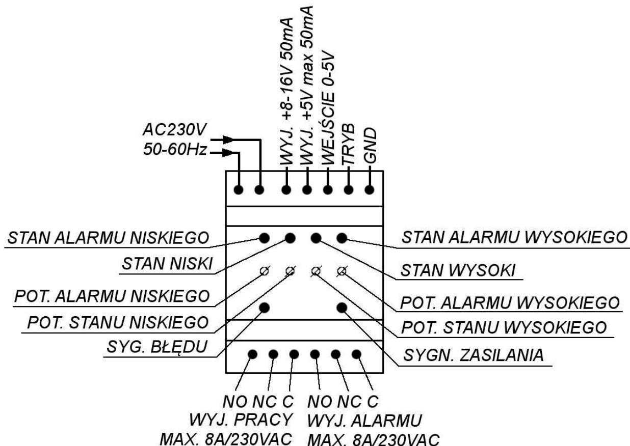
Rys. 1. Rozkład wyprowadzeń, elementów sygnalizacji i regulacji sterownika
