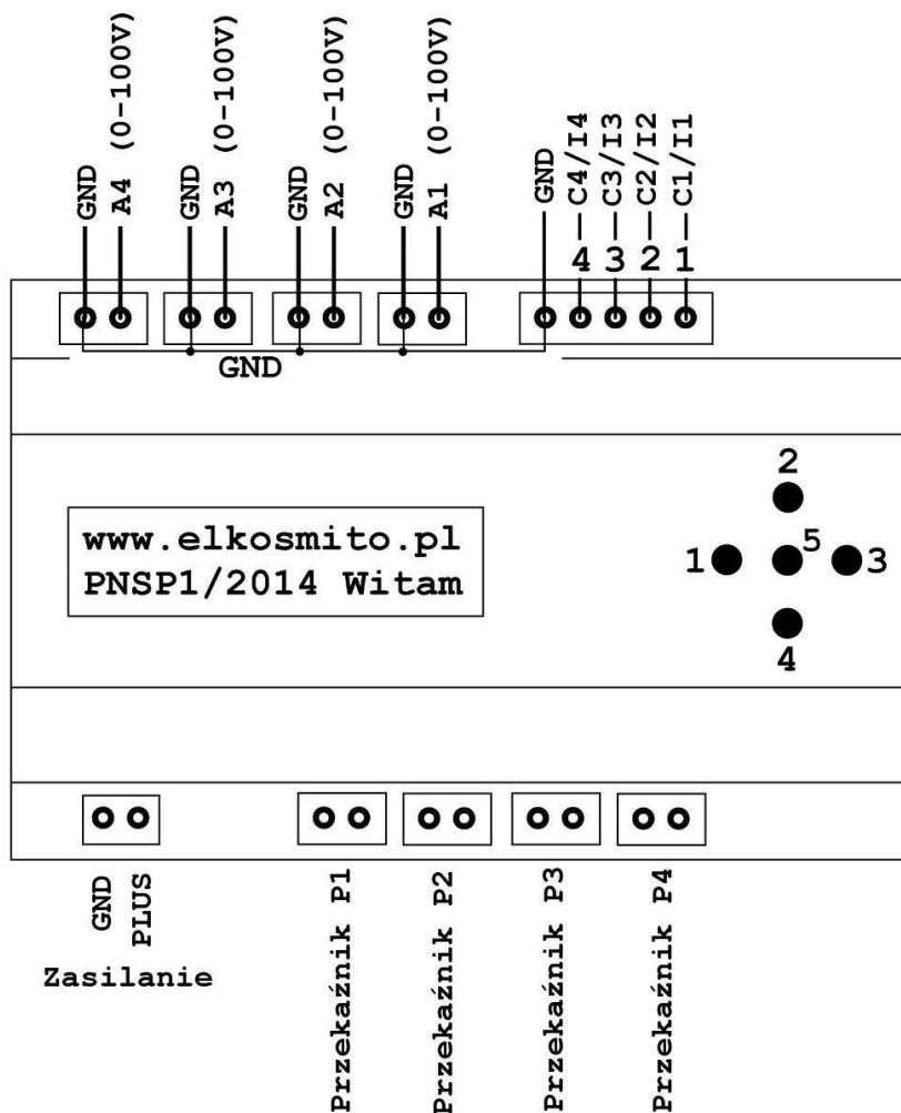
Rys. 1. Wyprowadzenia sterownika
