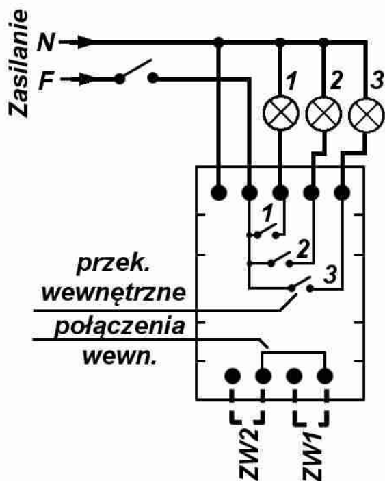
Rysunek 1: Podłączenie układu
