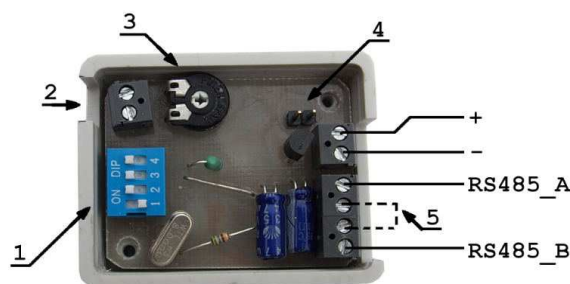
Rys. 1: Podłączenie modułu
